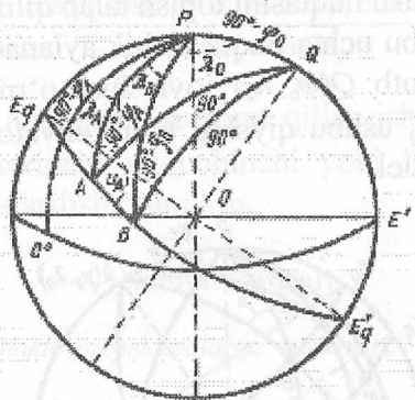
20-rasm. Berilgan ikkita nuqta (A, B) bo'yicha qiyshiq qutb koordinatalar tizimini hisoblash chizmasi
