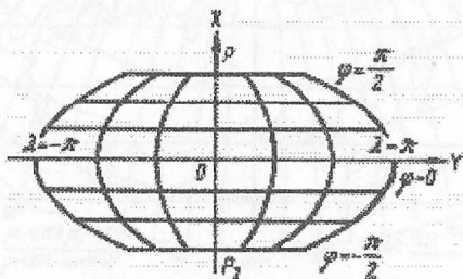
42-rasm. Psevdosilindrik proyeksiyalar koordinatalari tizimi
