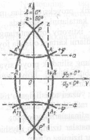
37-rasm. Ko'ndalang silindrik proyeksiyalarda koordinatalar tizimi
