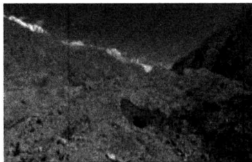
15.6-rasm. Tub (ostki) morenalar. http://www.segodnya.ua
