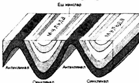
5.1-rasm. Antiklinal va sinklinal burmalar.
