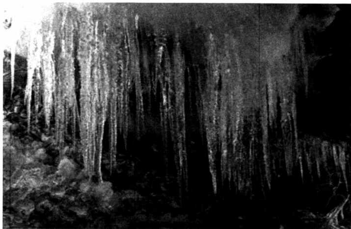
12.6- rasm. Karst g'oridagi stalaktitlar. www/Saga.ua
