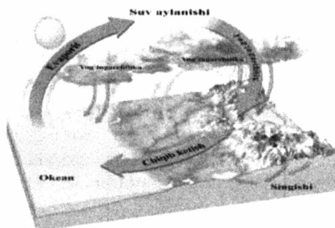
9.1-rasm. Yer yuzasidagi suv oqimlarining aylanishi.
