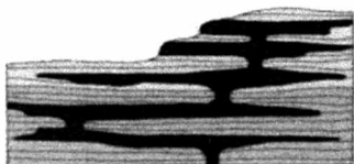
5.11-rasm. Ko'p yarusli sillar.
