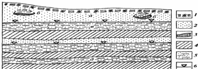
12.3-rasm. Yer po'stida turli erosti suvlarining joylashish sxemasi: a - sizot suvlari; b - verkhovodka; v - grunt suvlari; g, d - qatlam suvlari; 1 - tuproq-o'simlik qatlami; 2 - suv o'tkazuvchi qatlam; 3 - yarim suv o'tkazuvchi jinslar; 4 - suv o'tkazmaydigan qatlam; 5 - gravitatsion suv; 6 - grunt suvlarining sathi.
