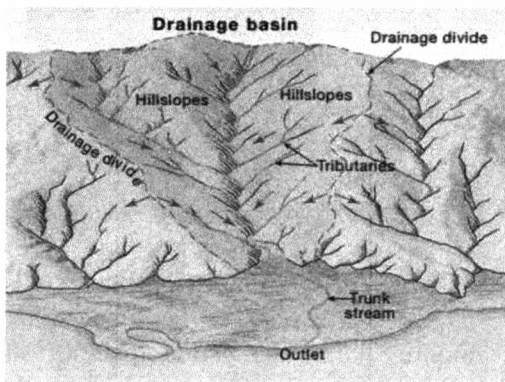
10.1- rasm. Daryo havzalarining suvayirg‘ichlari.
