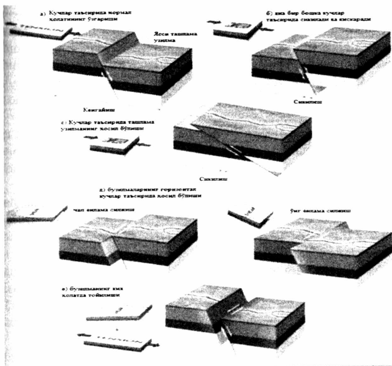
5.3-rasm. Tektonik kuchlar ta'sirida hosil bo'lgan buzilmalar.
