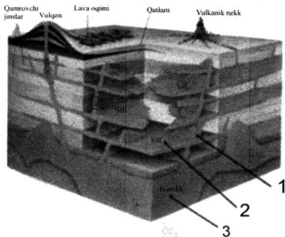
5.6-rasm. Magmatik jinslarning yotish shakllari. 1- dayka. 2- sill, 3- batolit. (Understanding Earth., J. Grotzinger, T. H. Jordan, F. Press, R. Siyever.)
