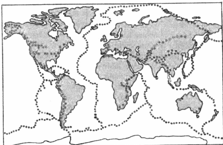
5.23-rasm. Yyer shari yuzasida seysmik mintaqalarning joylashishi
