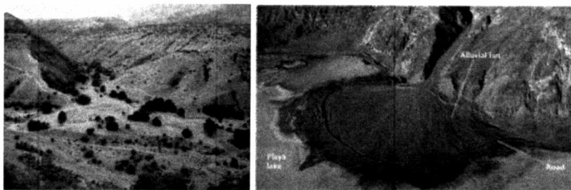
9.2-rasm. Chiqaruv konusi.
