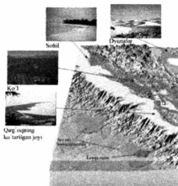
10.11-rasm. Estuariyning shakllanishi.
