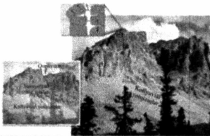
14.3- rasm. Tog' jinslarining muzlashi ta'sirida emirilishi
