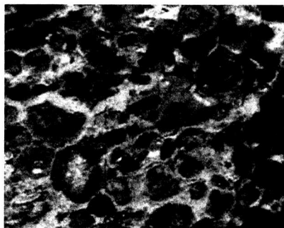
12.17-rasm. Terrarossa jinsi.
