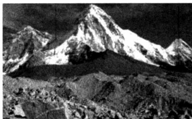
15.7-rasm. Oxirgi morena. http://www.segodnya.ua
