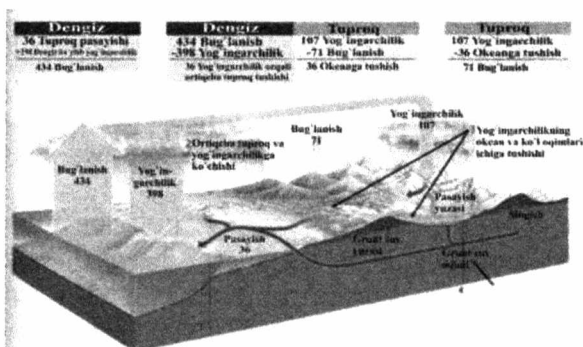
12.2-rasm. Yerning atmosfera, okean, ko'l va daryo suvlarining sirkulyasichsi.
