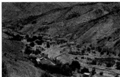
10.6-rasm. U shaklidagi vodi.
